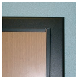
Vista interna dos perfis de remate e de fixação do revestimento interno na versão GRAFFA
